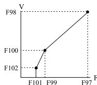
圖3 (高啟動轉矩)
