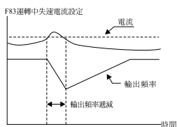
運轉中過電流失速防止功能
