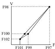
圖2 (風、水力機械)
