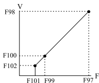
圖1 (一般用途)
