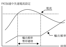
加速中過電流失速防止功能
